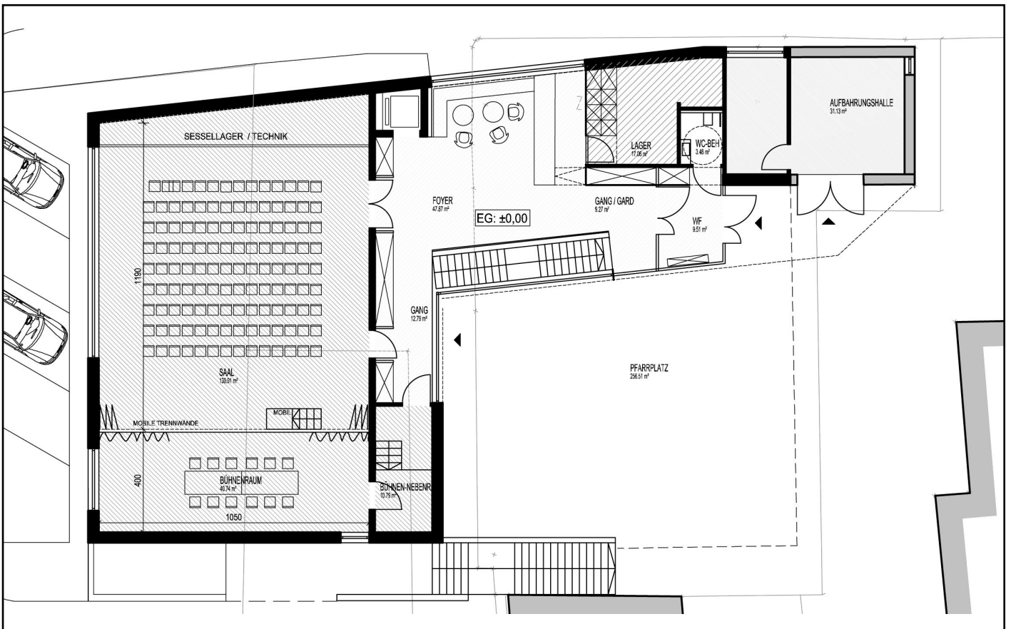
Erdgeschoß
